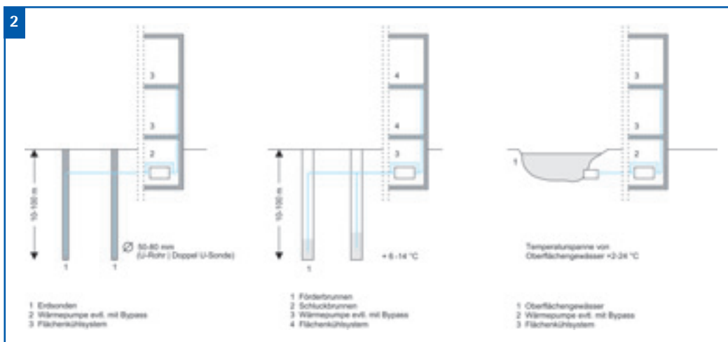
Abbildung 2 Nutzung verschiedener Wärmesenken (Erdsonden, Grundwasserbrunnen, Flusswasser) zur Kühlung durch Bauteilaktivierung Quelle: Institut für Entwerfen und Konstruieren, Leibniz Universität Hannover
